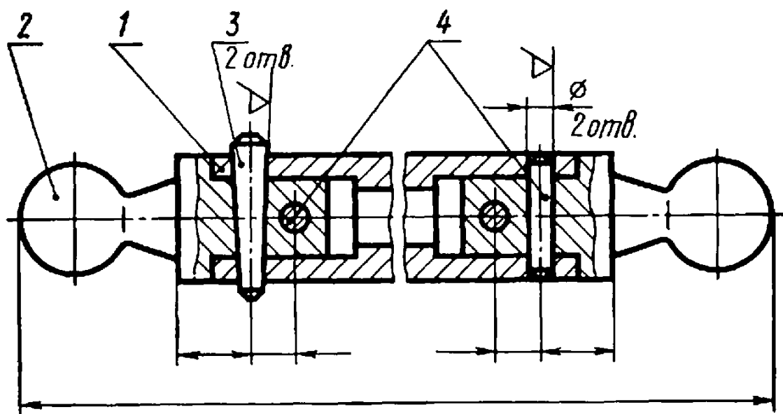
Сборочный чертеж
